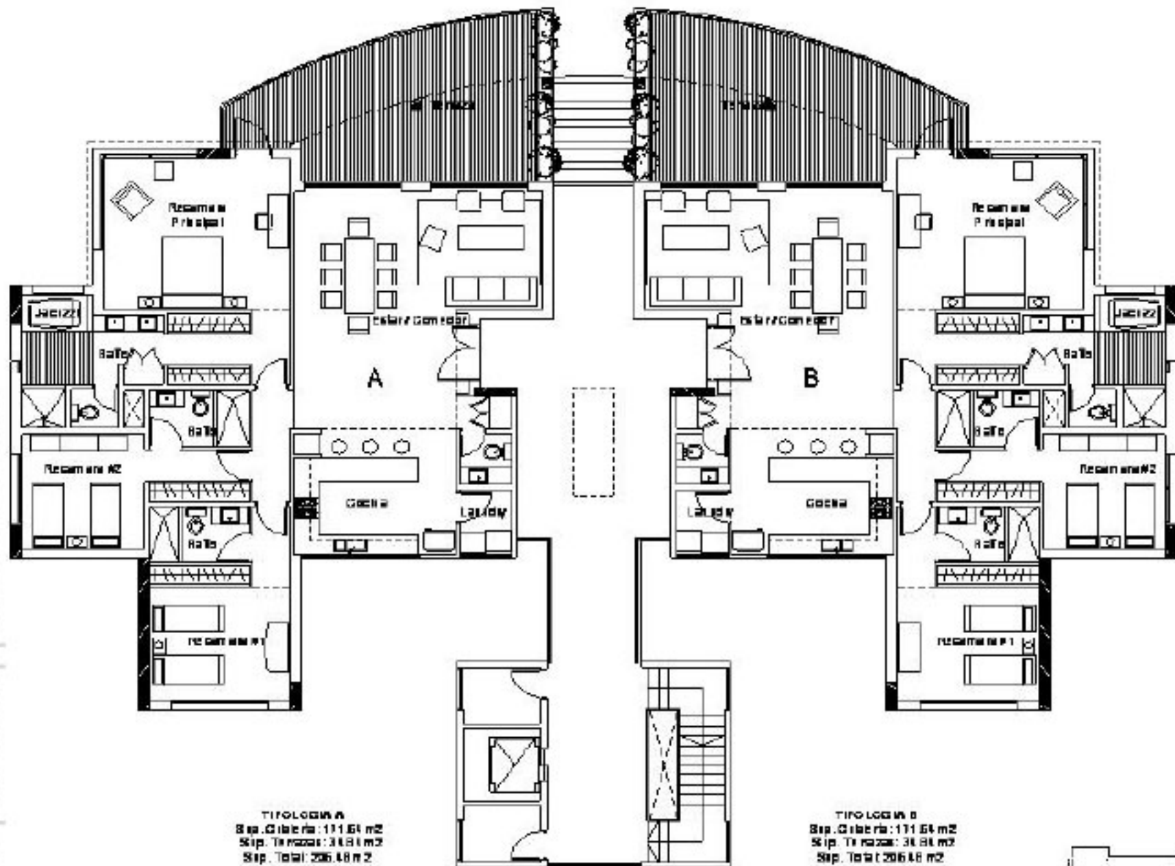
PLANTA AMOBLADA - NIVEL 01
